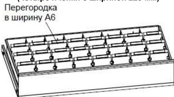
7xКД-516/536 Перегородка в глубину +24xКД-516/536 Перегородка в ширину CD (восемь ячеек с шириной 115 мм)
